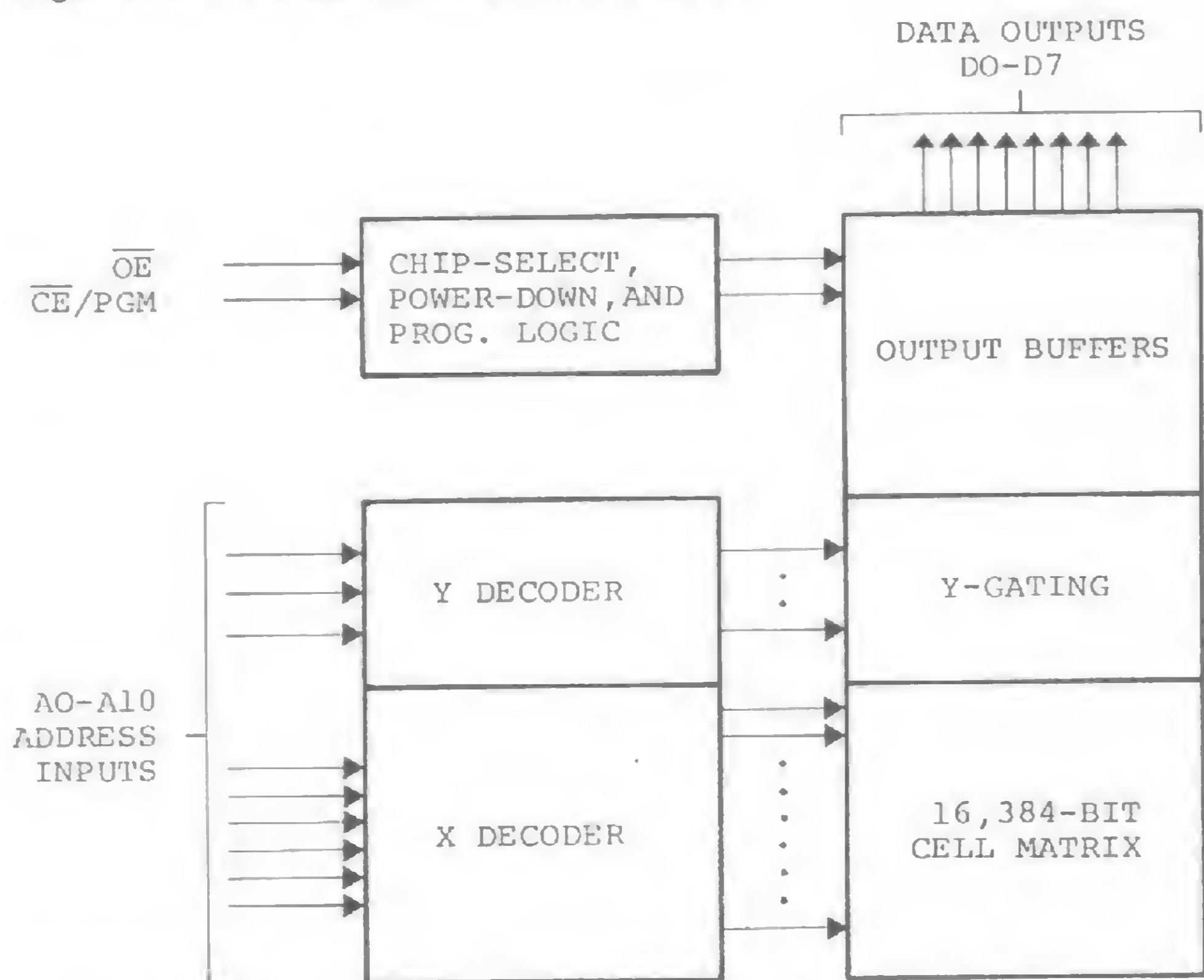
Figura B – Diagrama de blocos da EPROM 2716
